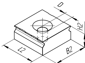
Ultra Spannkrallen
