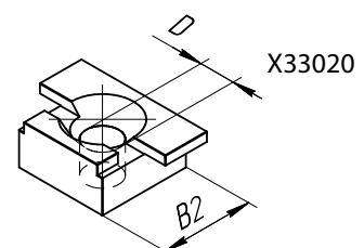
Klemmbacken Anschlag
